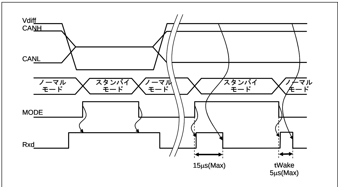
図 5 モード切り替え時の RxD
